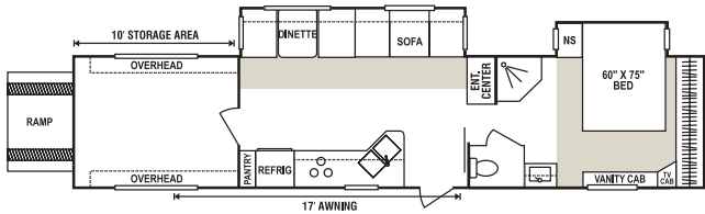
37Px2 • UVW 11500 • Dry Hitch Wt. 2400 • NCC 2500 • Length 39'2"
