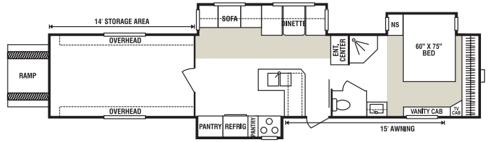
41Kx2 • UVW 13200 • Dry Hitch Wt. 3220 • NCC 5200 • Length 43'3"
