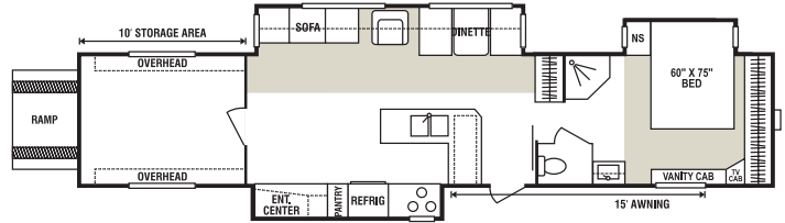
41KGx2 • UVW 14140 • Dry Hitch Wt. 3060 • NCC 3860 • Length 43'8"
