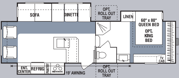
305KS3 • UVW 8796 • Dry Hitch Wt. 2021 • NCC 1204 • Length 32'2"
