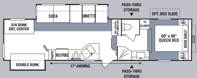
325BH • UVW 8770 • Dry Hitch Wt. 1590 • NCC 1730 • Length 33'5"
