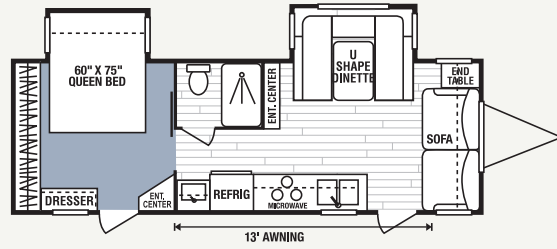
260FL • UVW 5224 • Dry Hitch Wt. 799 • NCC 1776 • Length 28'10"
