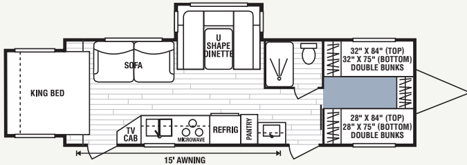
289KS • UVW 5028 • Dry Hitch Wt. 450 • NCC 1972 • Length 30'6"
