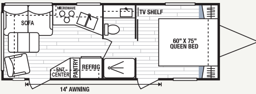
240RL • UVW 3819 • Dry Hitch Wt. 584 • NCC 1681 • Length 26' 5"
