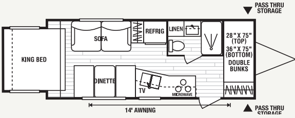
210KS • UVW 3821 • Dry Hitch Wt. 460 • NCC 1679 • Length 23'4"
