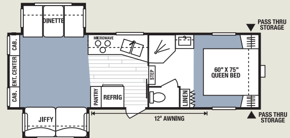
265RLS • UVW 5845 • Dry Hitch Wt. 879 • NCC 1655 • Length 28'2"
