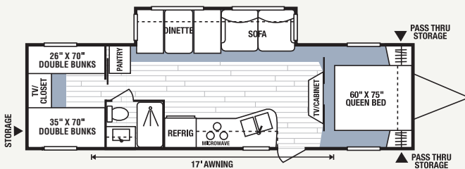
324BHS • UVW 5570 • Dry Hitch Wt. 653 • NCC 1930 • Length 33'7"
