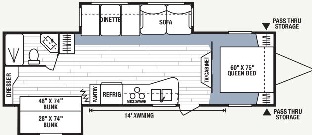
318BHS • UVW 5577 • Dry Hitch Wt. 708 • NCC 1923 • Length 32'9"
