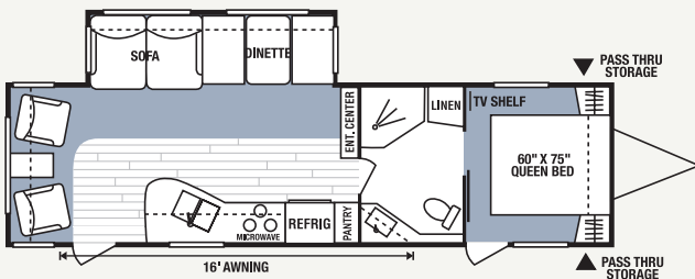
323RLS • UVW 5357 • Dry Hitch Wt. 558 • NCC 2143 • Length 32'1"
