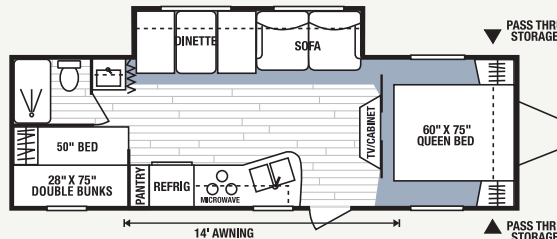
290BHS • UVW 5450 • Dry Hitch Wt. 639 • NCC 1550 • Length 31'3"
