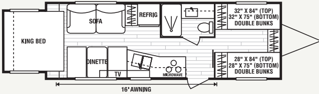
255KS • UVW 4474 • Dry Hitch Wt. 504 • NCC 2026 • Length 28'1"
