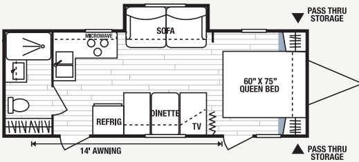
240RBS • UVW 4242 • Dry Hitch Wt. 432 • NCC 1758 • Length 26'9"
