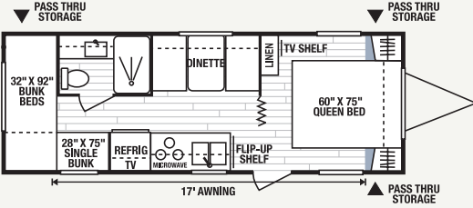
240BH • UVW 4169 • Dry Hitch Wt. 509 • NCC 1831 • Length 26'9"
