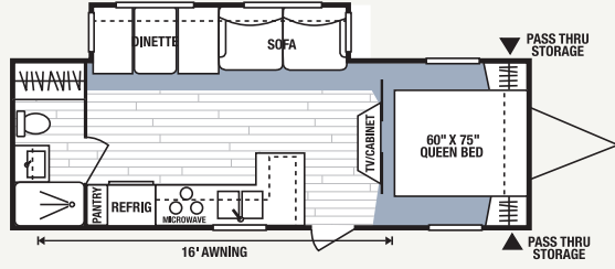
260RBS • UVW 5057 • Dry Hitch Wt. 552 • NCC 1743 • Length 28'8"
