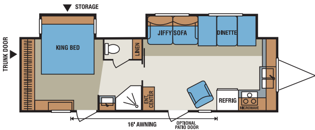
S310FK • UVW 7,300 • Dry Hitch Wt. 1,250 • NCC 1,500 • Length 33'9"
