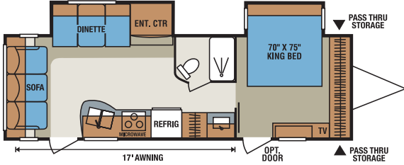
S290KB • UVW 6,590 • Dry Hitch Wt. 740 • NCC 2,210 • Length 33'10"
