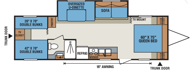
S314BH • UVW 5,600 • Dry Hitch Wt. 550 • NCC 1,620 • Length 32'8"
