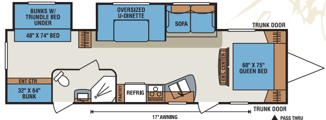
S321BH • UVW 7,010 • Dry Hitch Wt. 730 • NCC 1,790 • Length 34'6"
