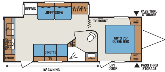
S261RK • UVW 4,970 • Dry Hitch Wt. 380 • NCC 2,030 • Length 28'7"
