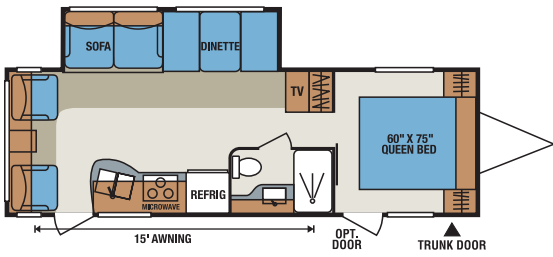
S280RL • UVW 5,110 • Dry Hitch Wt. 530 • NCC 1,890 • Length 29'7"
