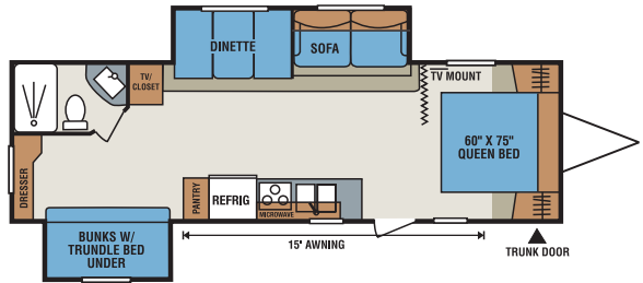
S318BH • UVW 5,800 • Dry Hitch Wt. 480 • NCC 1,420 • Length 31'11"
