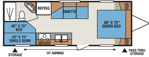
S242BH • UVW 3,910 • Dry Hitch Wt. 450 • NCC 2,090 • Length 26'6"
