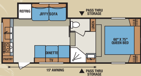
S235RK • UVW 5,810 • Dry Hitch Wt. 800 • NCC 1,990 • Length 25'3"
