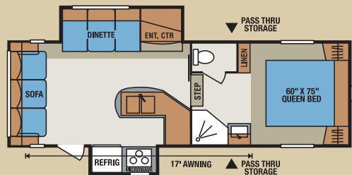
S245RL2 • UVW 6,680 • Dry Hitch Wt. 1,160 • NCC 2,120 • Length 27'6"
