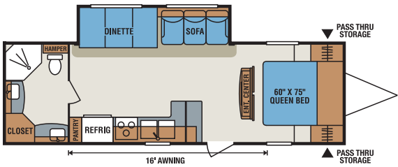
S290RBS • UVW 5,180 • Dry Hitch Wt. 560 • NCC 1,820 • Length 30'6"
