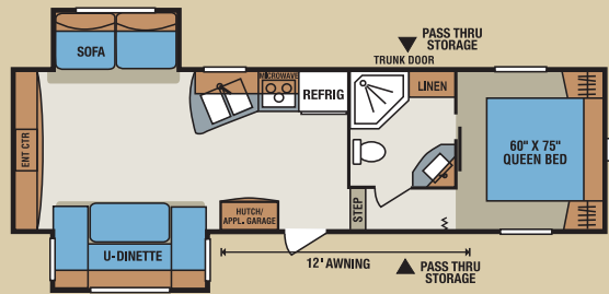
S265RE • UVW 7,050 • Dry Hitch Wt. 1,510 • NCC 1,950 • Length 30'9"
