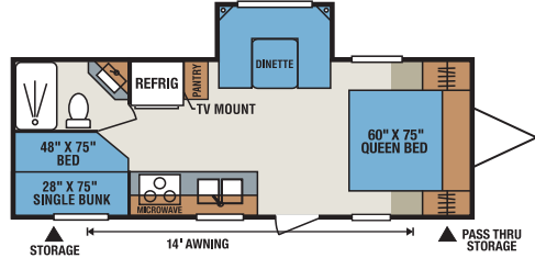
S242SBH • UVW 4,300 • Dry Hitch Wt. 540 • NCC 1,700 • Length 26'6"
