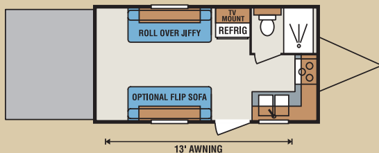
17TH • UVW 3,410 • Dry Hitch Wt. 640 • NCC 2,590 • Length 19'5.5"
