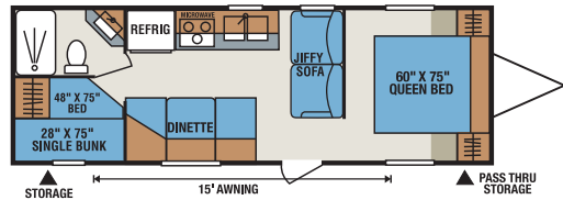
S272BH • UVW 4,290 • Dry Hitch Wt. 480 • NCC 2,710 • Length 30'
