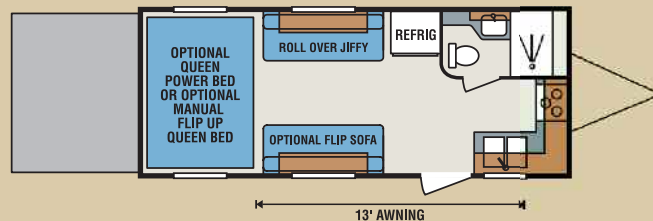
22TH • UVW 4,130 • Dry Hitch Wt. 820 • NCC 2,870 • Length 24'5.5"
