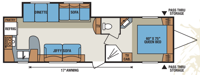
S310RKS • UVW 6,560 • Dry Hitch Wt. 550 • NCC 2,240 • Length 33'9"
