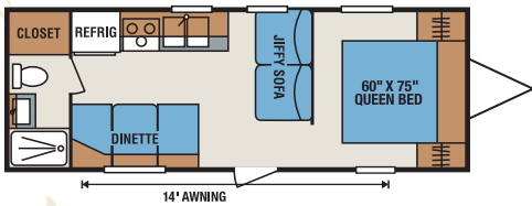
S240FB • UVW 4,010 • Dry Hitch Wt. 390 • NCC 1,990 • Length 26'3"
