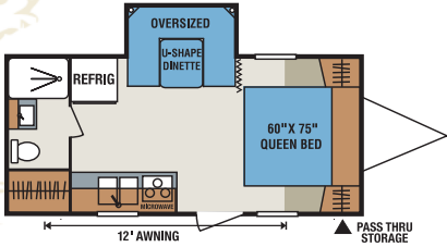
S202SRB • UVW 3,730 • Dry Hitch Wt. 430 • NCC 1,270 • Length 22'5"
