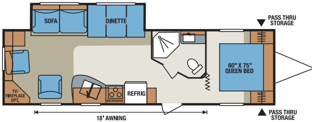
S290RE • UVW 5,700 • Dry Hitch Wt. 520 • NCC 1,900 • Length 32'6"
