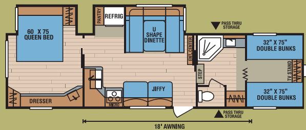
305BHS • UVW 7,340 • Dry Hitch Wt. 1,230 • NCC 1,460 • Length 33'10"
