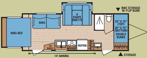
245KS • UVW 4,700 • Dry Hitch Wt. 530 • NCC 1,800 • Length 26'2"
