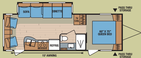
280RLS • UVW 5,210 • Dry Hitch Wt. 620 • NCC 1,790 • Length 29'9"
