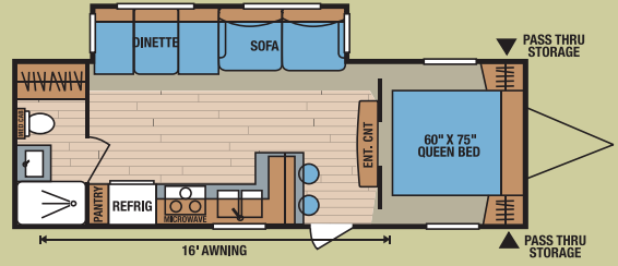
260RBS • UVW 5,040 • Dry Hitch Wt. 500 • NCC 1760 • Length 28'8"
