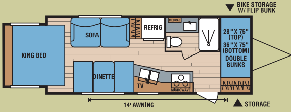
210KS • UVW 4,160 • Dry Hitch Wt. 490 • NCC 1,340 • Length 23'4"
