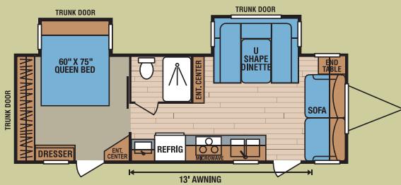
260FL • UVW 5,400 • Dry Hitch Wt. 870 • NCC 1,400 • Length 28'10"
