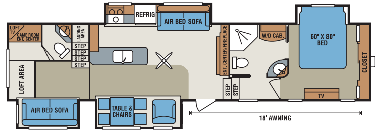
37RB • UVW 12,090 • Dry Hitch Wt. 1,920 • NCC 1,910 • Length 40'8"
