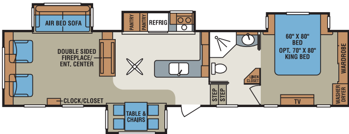
38CF • UVW 11,140 • Dry Hitch Wt. 2,260 • NCC 2,860 • Length 40'6"
