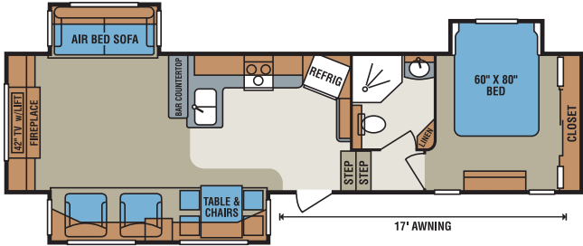
35RE • UVW 10,520 • Dry Hitch Wt. 2,000 • NCC 3,480 • Length 36'9"
