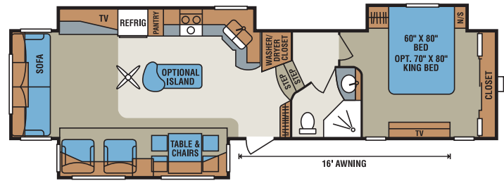
38SR • UVW 11,390 • Dry Hitch Wt. 2,110 • NCC 2,610 • Length 39'10"
