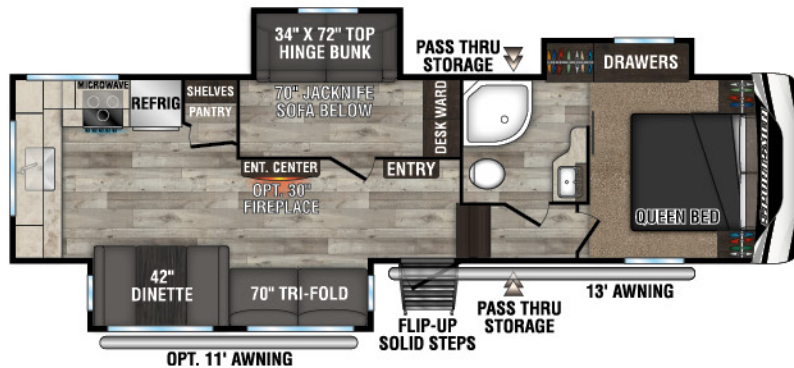
303MB UWW - 8,720 Exterior Length - 34'2" Sleeps - 7
