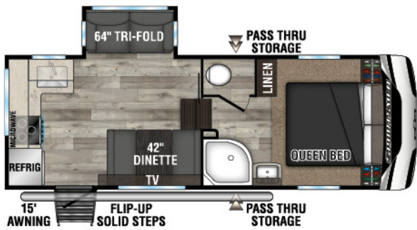
231RK UWW - 6,200 | Exterior Length - 24'10" | Sleeps - 5
