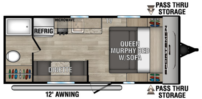
170MB UYW - 2,980 | Exterior Length - 22' | Sleeps - 3
